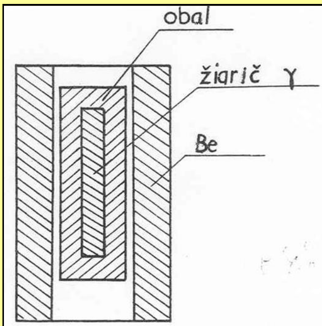
Obr. 10.3 Schematické zobrazenie konštrukcie ( \gamma , n) zdroja s vynímateľným \gamma -žiaričom
