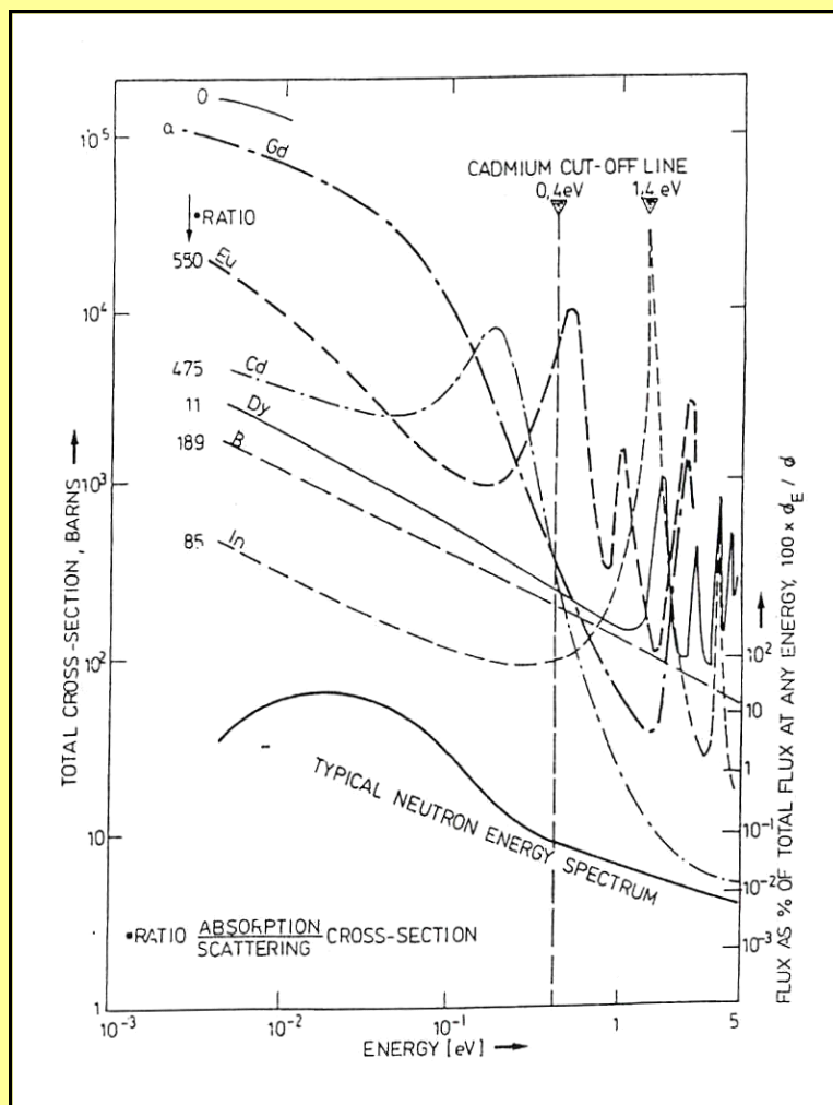
Závislosť celkového účinného prierezu od energie
